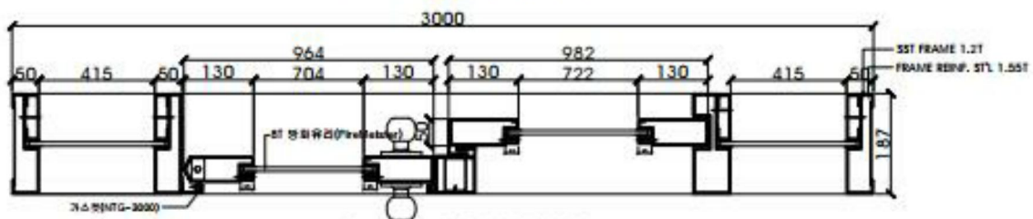
A-2 SECTION
