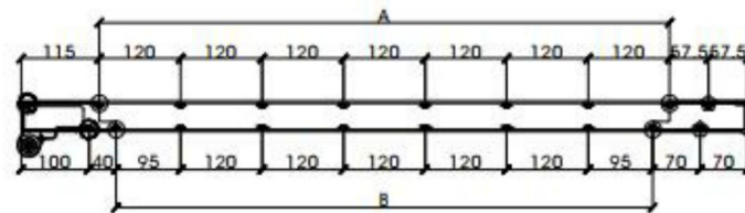
A-2 SECTION
