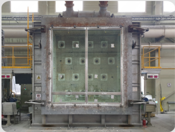
120분 내화구조(유리벽체)
